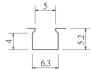
溝槽尺寸
