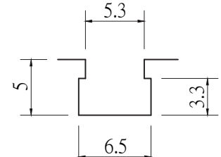
溝槽尺寸
